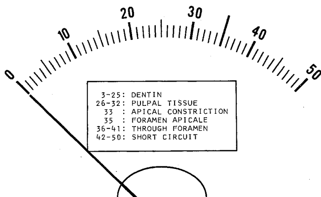
Fig. 8. Skalaen på analoge apparater kan indeledes efter vævsområde. Electronic Apex Control®.
