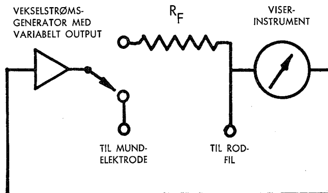
Fig. 6. Den elektriske principskitse for apparat med analog aflæsning.
