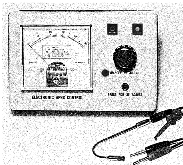
Fig. 5. Instrument med analog aflæsning, Electronic Apex Control®.
