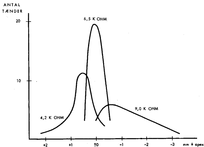
Fig. 7. Ved forskellige modstandsværdier registreres rodmål i varierende afstand fra vertex.
