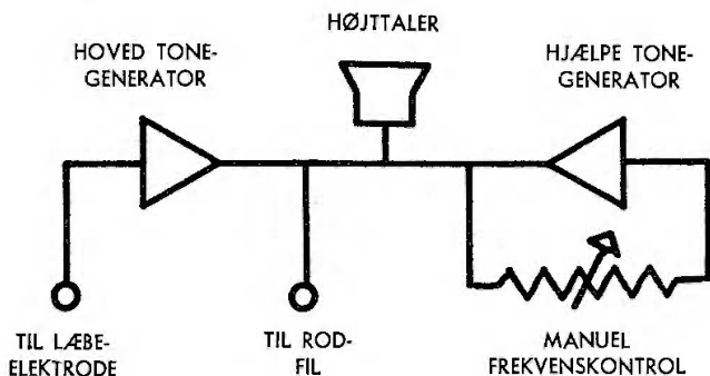
Fig. 10. Den elektriske principskitse for et apparat med audio-visuel indikation.
